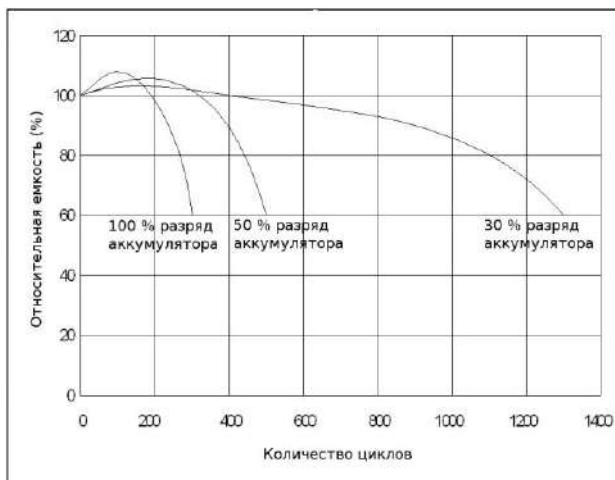
Зависимость рабочих характеристик аккумулятора от глубины разряда
