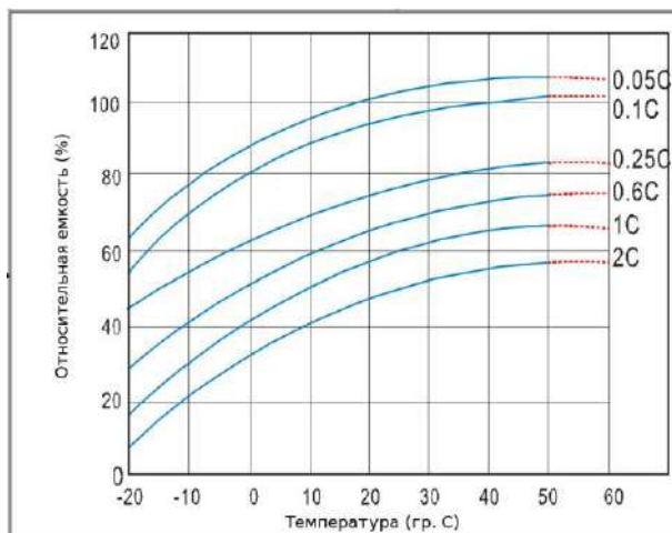
Зависимость емкости от температуры
